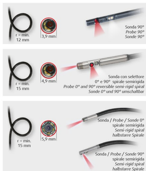
Sonda MASTER, spirale semirigida MASTER probes, semi-rigid spiral MASTER Sonden, halbstarre Spirale
